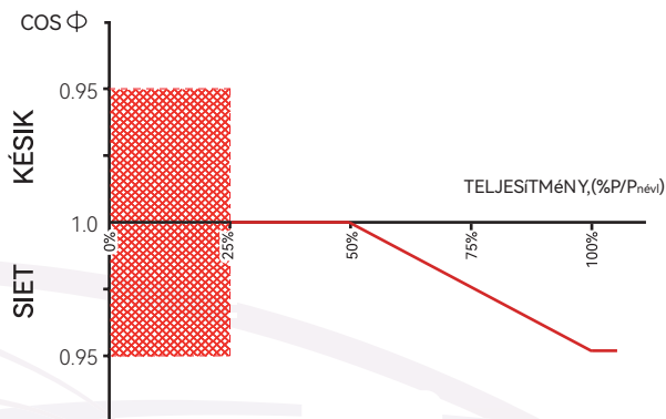
7-2. ábra Q(P) görbe
