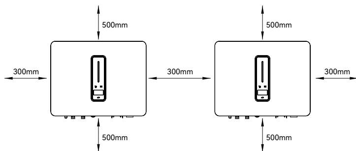
4-2. ábra Ajánlott beépítési térköz
