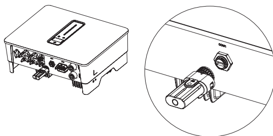
5-10. ábra A felügyeleti eszköz telepítése
